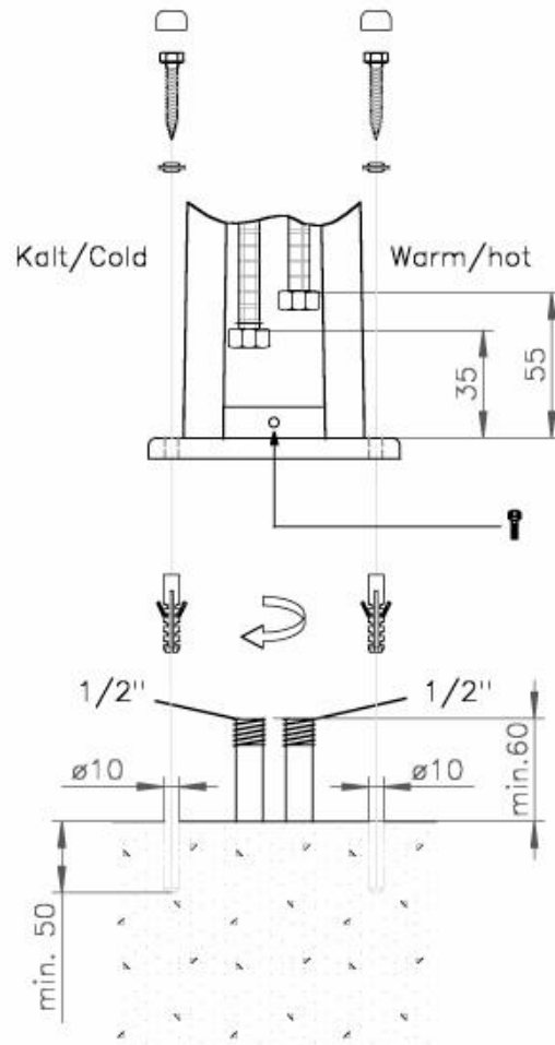
Ansicht A / view A
